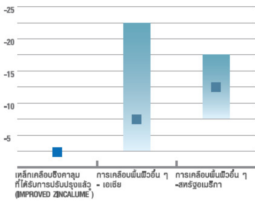
การเปลี่ยนแปลงของสีโมโนเคลที่แตกต่างกัน บริเวณที่ร้อนและเย็นของแผ่นเหล็ก
